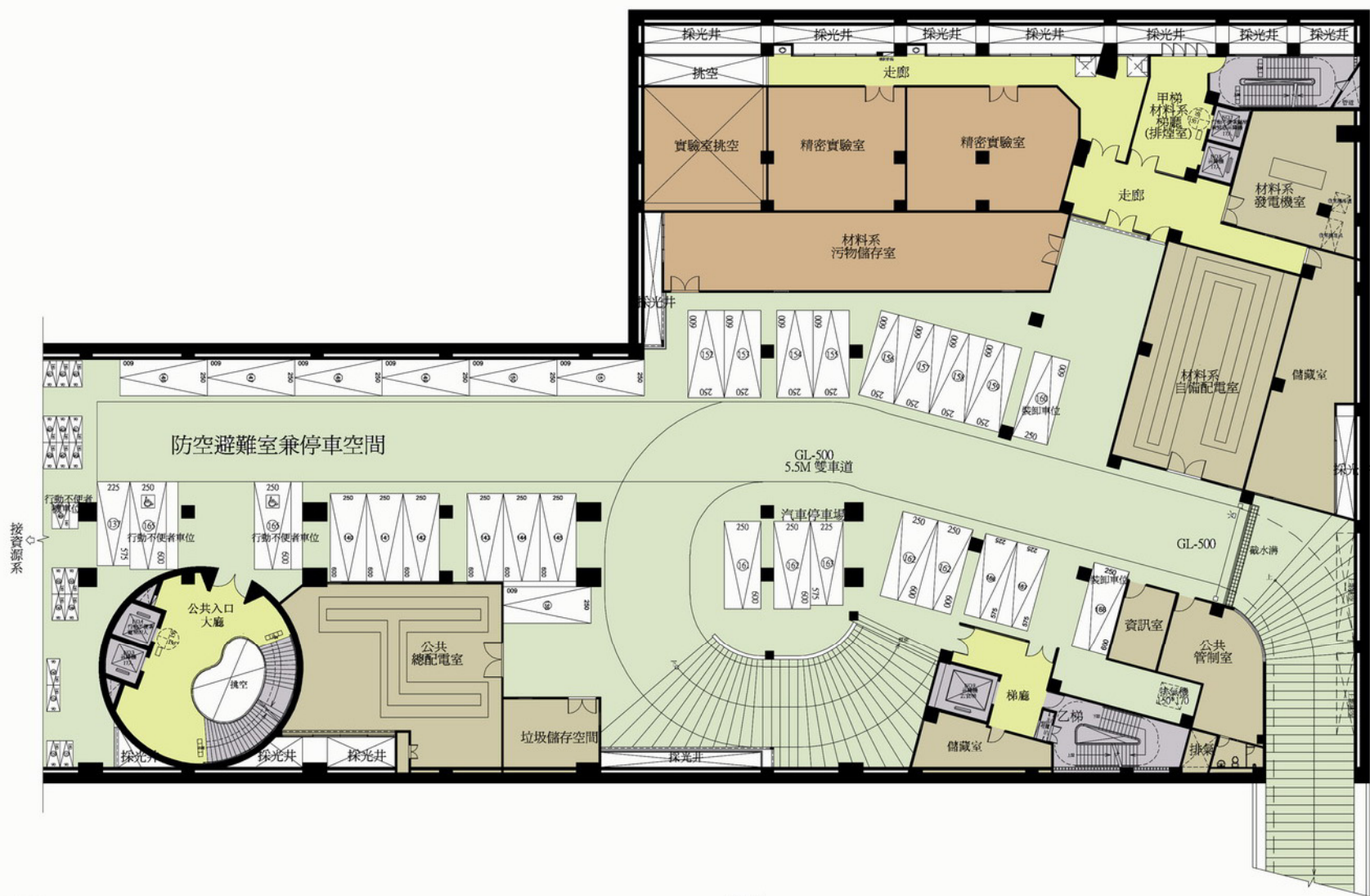
材料系地下一層平面圖
