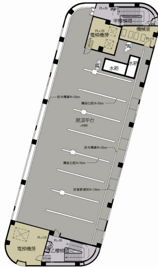
材料系屋頂層平面圖
