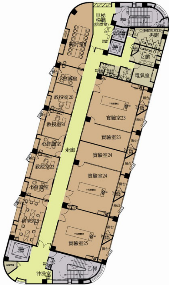
材料系九層平面圖
