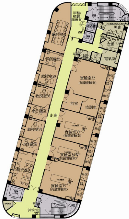
材料系十二層平面圖
