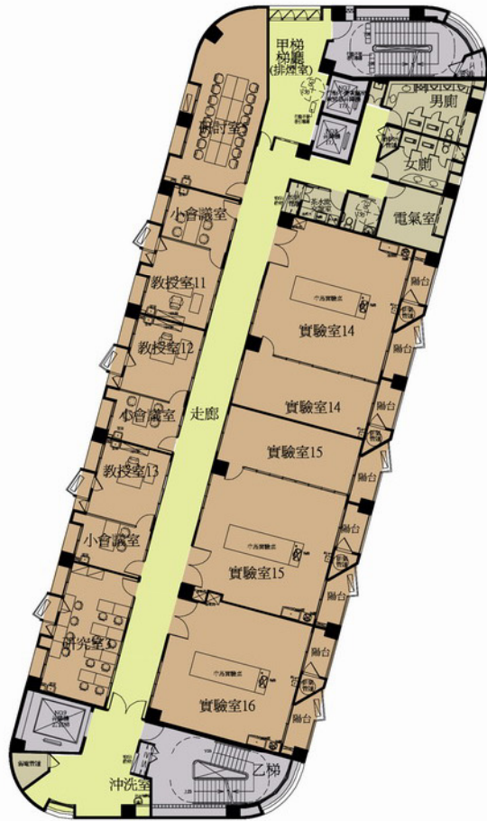
材料系六層平面圖
